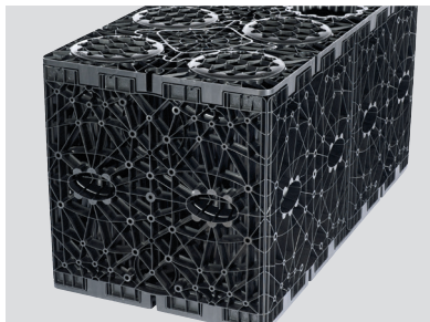
Rigolensystem ACO Stormbrixx
