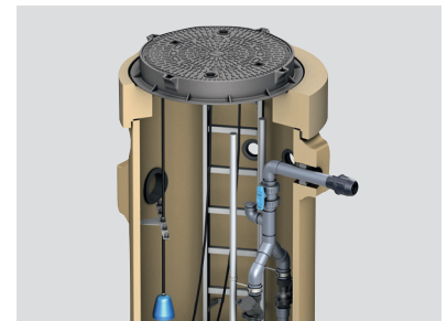
ACO Pumpstation Powerlift im Polymerbetonbehälter
